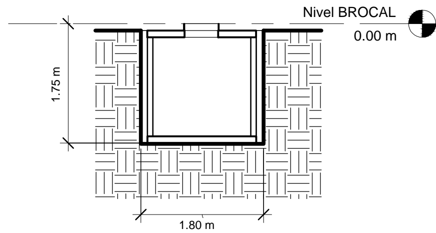
4 Sección 0 1 : 50
