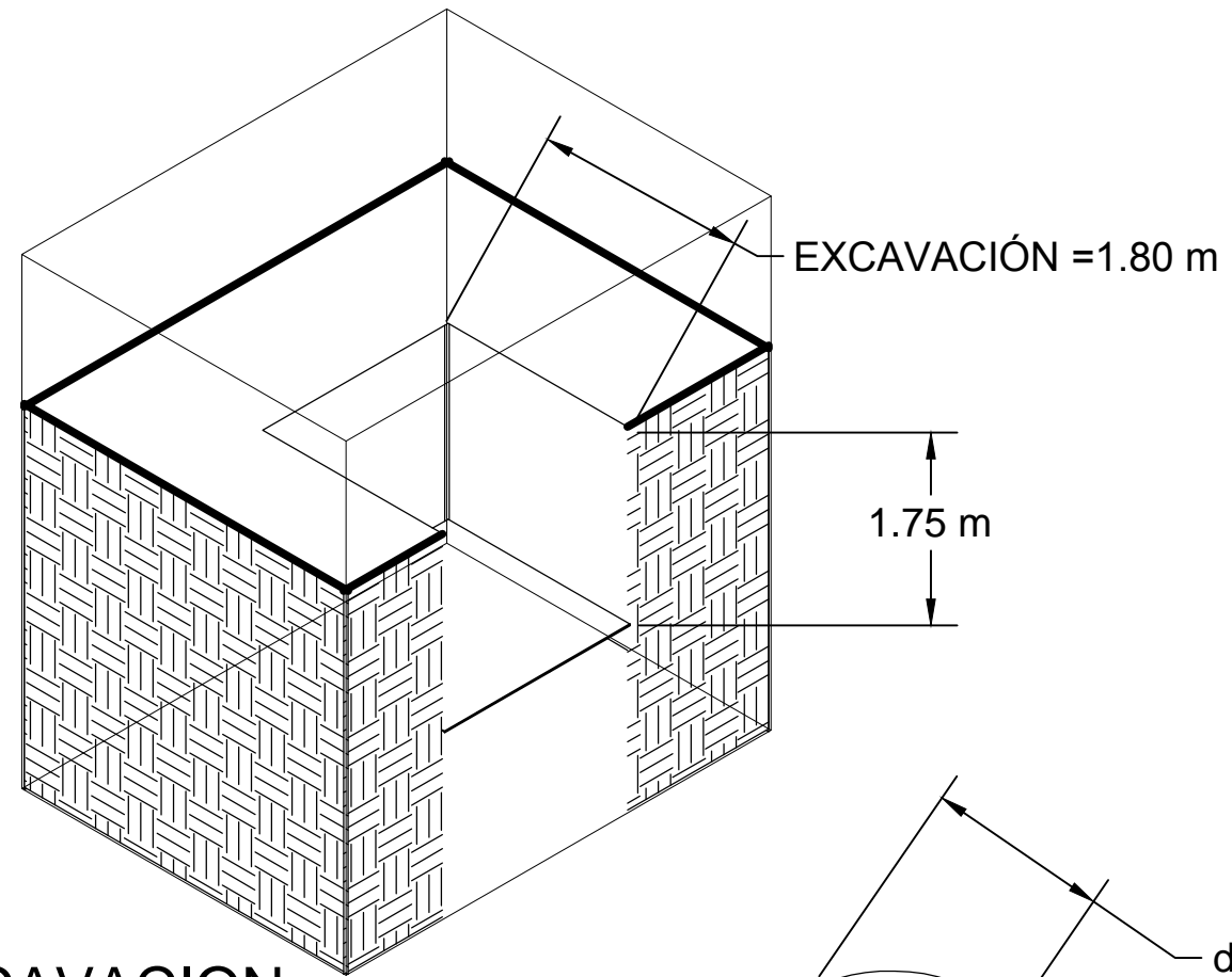
1 EXCAVACION
